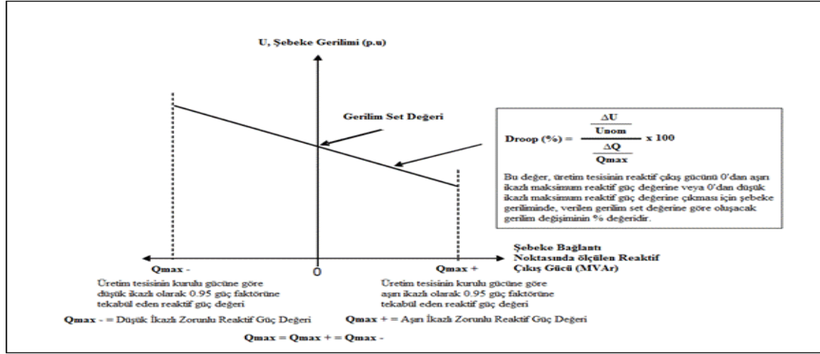
Şekil E.18.6 Üretim Tesisleri Tarafından Sisteme Verilecek Reaktif Güç Destegi Eğrisi
