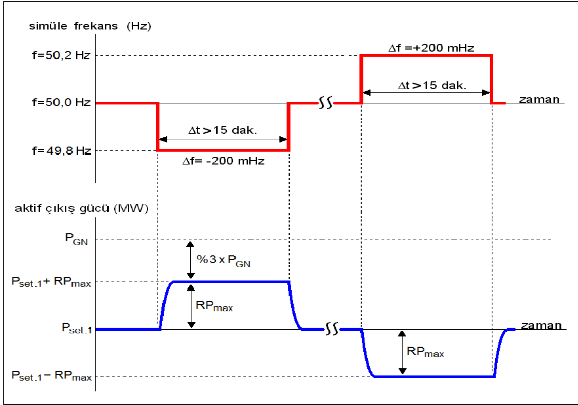
Şekil-E.17.A.2. Maksimum çıkış gücü seviyesi için Primer Frekans Kontrol Rezerv Testi Simule Frekans Uygulanışı
