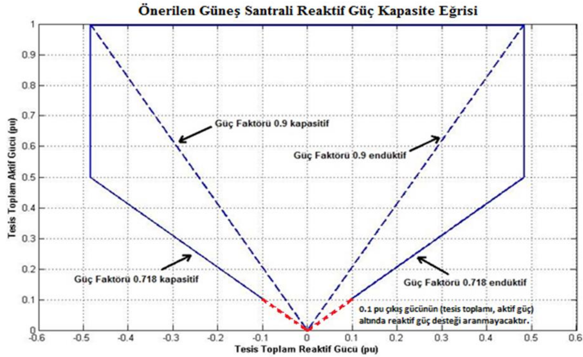
Şekil E.18.3 Rüzgar Santrali Reaktif Güç Kapasite Eğrisi
