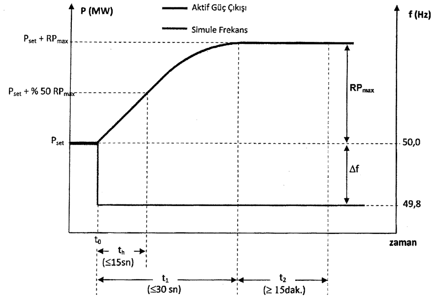
Şekil E.17.A.4 - f=49,8 Hz'lik Simule Frekans Uygulamasında Üniteden Beklenen Tepki
