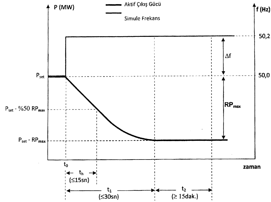
Şekil E.17.A.5 - f=50,2 Hz'lik Simule Frekans Uygulamasında Üniteden Beklenen Tepki
