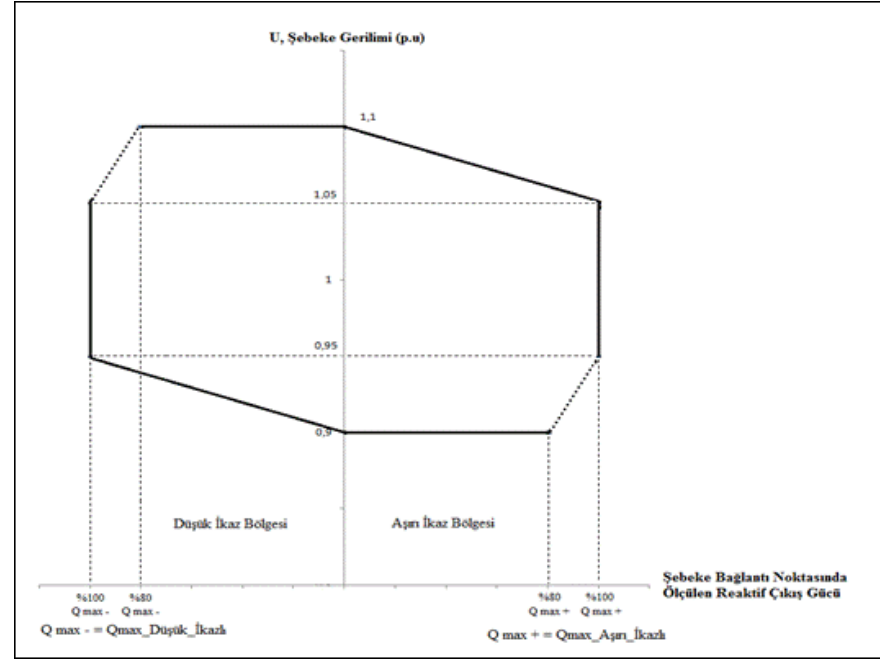
Şekil E.18.5 Zorunlu Reaktif Güç Değerlerinin Bağlantı Noktası Gerilimine Bağlı Değişimi
