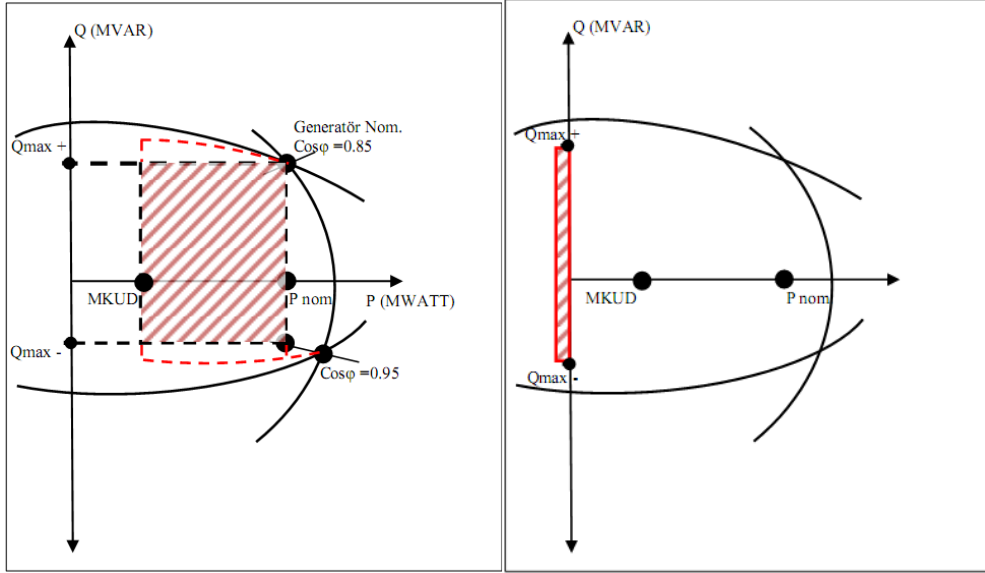
Şekil E.17.C.1.1 – Test Hedeflerinin Karşılandığı Durumlar (Jeneratör)
