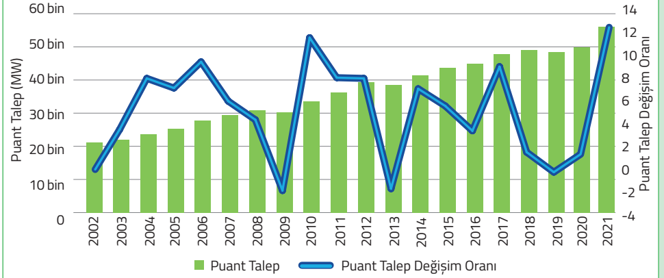
Puant Talep ve Değişim Oranı (MW-%)
